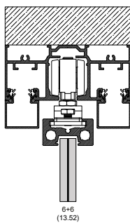
sliding door
