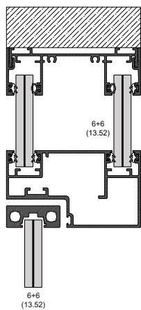
door & skylight
