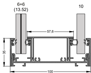
sliding door
